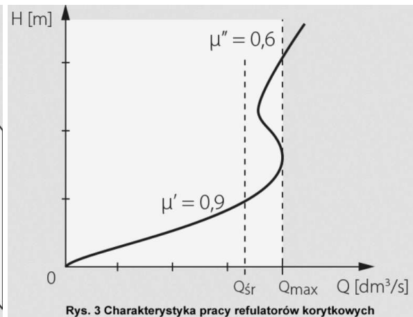
Rys. 3 Charakterystyka pracy refulatorów korytkowych
